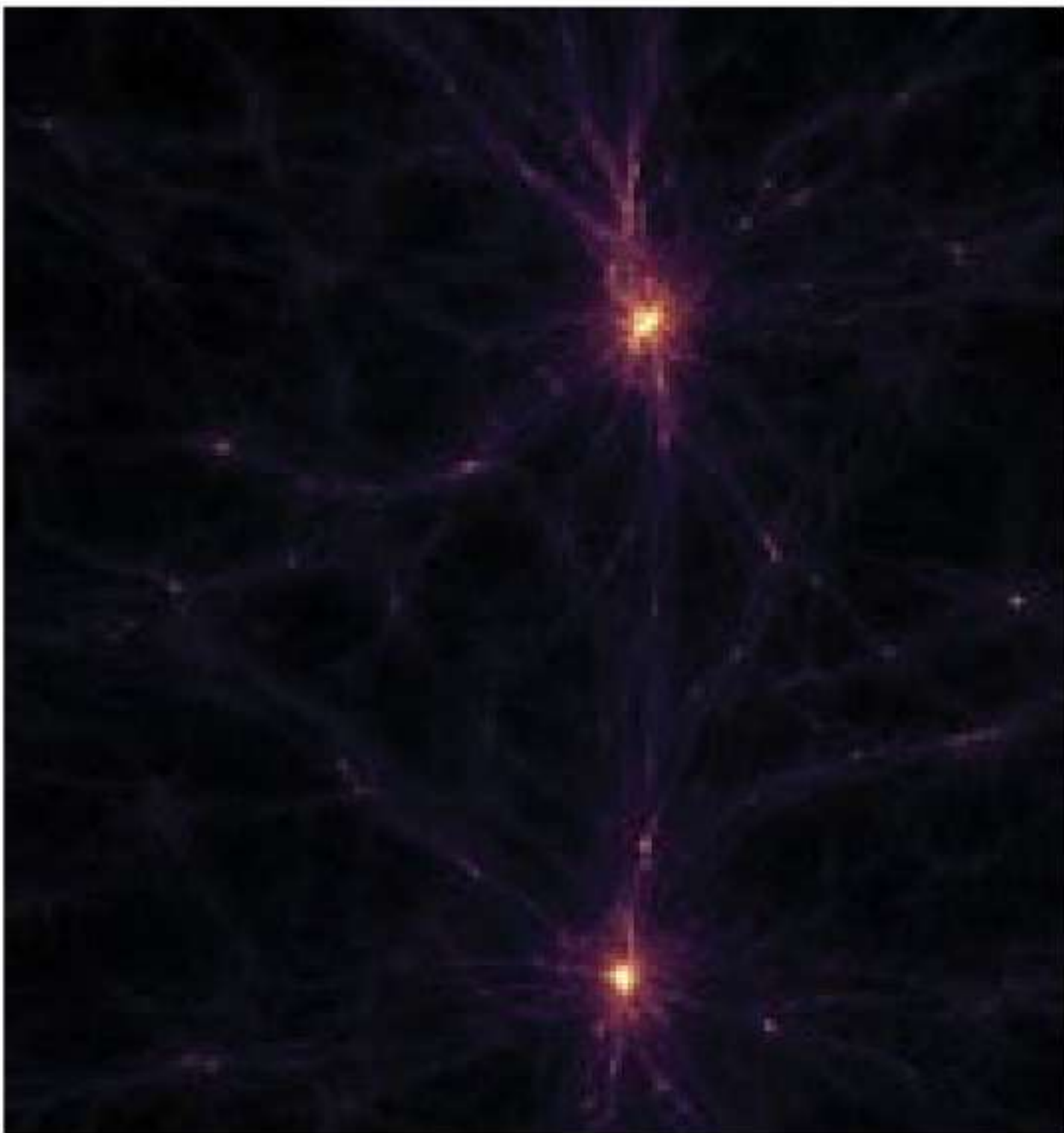
Galaxias
